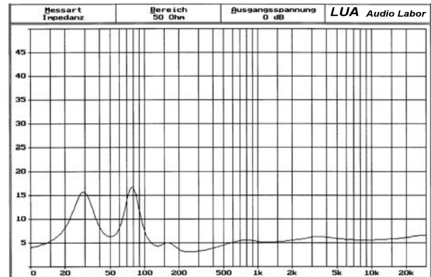
Lautsprecher: Impedanzkurve
