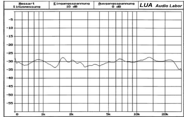
Frequenzgang: Mittel- Hochtonbereich
